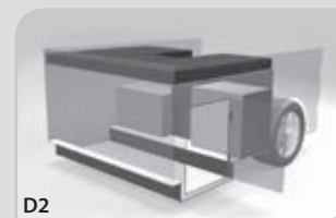
D2 Garaje debajo de camas individuales con prolongación chasis rebajada
