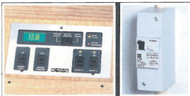
Het bedienings- en controlepaneel van de transformator/acculader.
